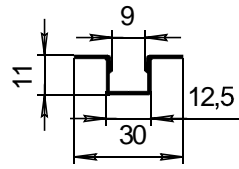
СПЛ-14-203 Прижим J_x=0,09\text{см}^4 J_y=0,3\text{см}^4
