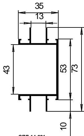
СПЛ-14-201 Ригель J_x=13,75\text{см}^4 J_y=3,54\text{см}^4
