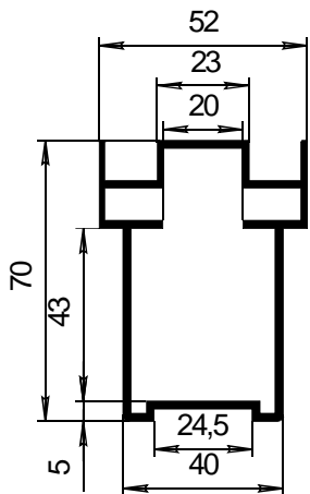
СПЛ-14-005 Элемент створки J_x=30,0\text{см}^4 J_y=16,22\text{см}^4
