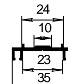
СПЛ-14-210 Нижний притвор створки J_x=0,05\text{см}^4 J_y=1,45\text{см}^4
