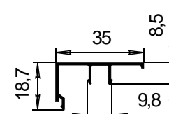
СПЛ-14-211 Вертикальный притвор створки J_x=0,3\text{см}^4 J_y=2,25\text{см}^4
