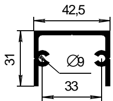
СПЛ-14-202 Сухарь J_x=2,62\text{см}^4 J_y=8,73\text{см}^4
