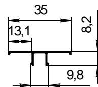
СПЛ-14-204 Штапик J_x=0,02\text{см}^4 J_y=0,45\text{см}^4
