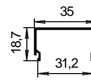
СПЛ-14-207 Штапик J_x=0,33\text{см}^4 J_y=1,72\text{см}^4
