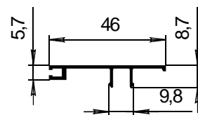
СПЛ-14-205 Штапик J_x=0,04\text{см}^4 J_y=1,6\text{см}^4
