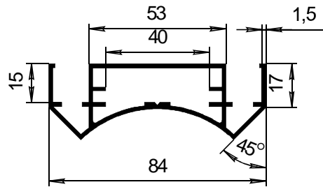
СПЛ-14-002 Поворотный элемент стойки J_x=3,17\text{см}^4 J_y=28,75\text{см}^4
