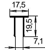
СПЛ-14-206 Крышка стойки СПЛ-14-004 J_x=0,27\text{см}^4 J_y=0,14\text{см}^4
