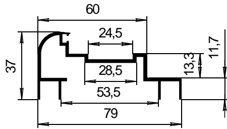
СПЛ-14-209 Профиль рамный J_x=2,65\text{см}^4 J_y=21,1\text{см}^4
