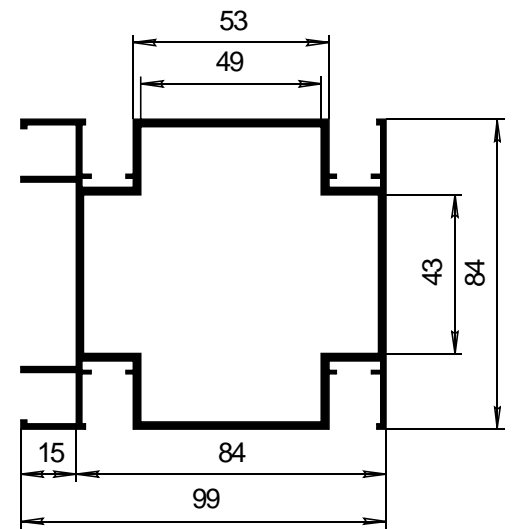
СПЛ-14-004 Стойка 3-х сторонняя J_x=84,62\text{см}^4 J_y=101,5\text{см}^4
