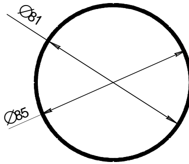
СПЛ-14-003 Стойка поворотная J_x=44,76\text{см}^4 J_y=44,76\text{см}^4
