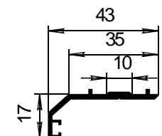
СПЛ-14-211 Вертикальный притвор створки J_x=0,3\text{см}^4 J_y=2,25\text{см}^4
