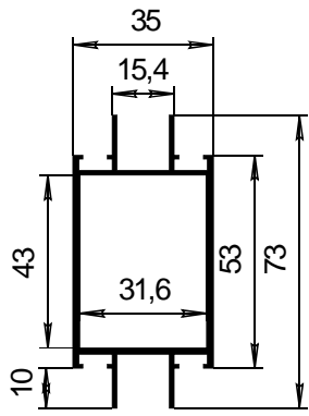
СПЛ-14-001 Стойка-ригель J_x=14,88\text{см}^4 J_y=6,13\text{см}^4
